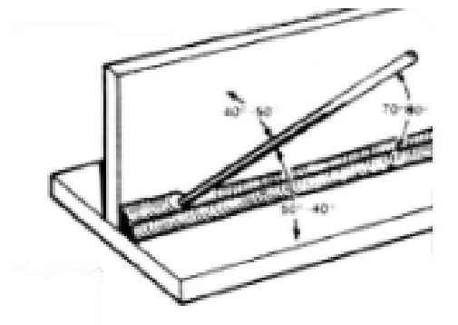
(Gambar sudut arah pengelasan)
