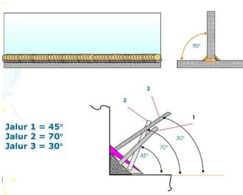
(Gambar sudut elektroda)
